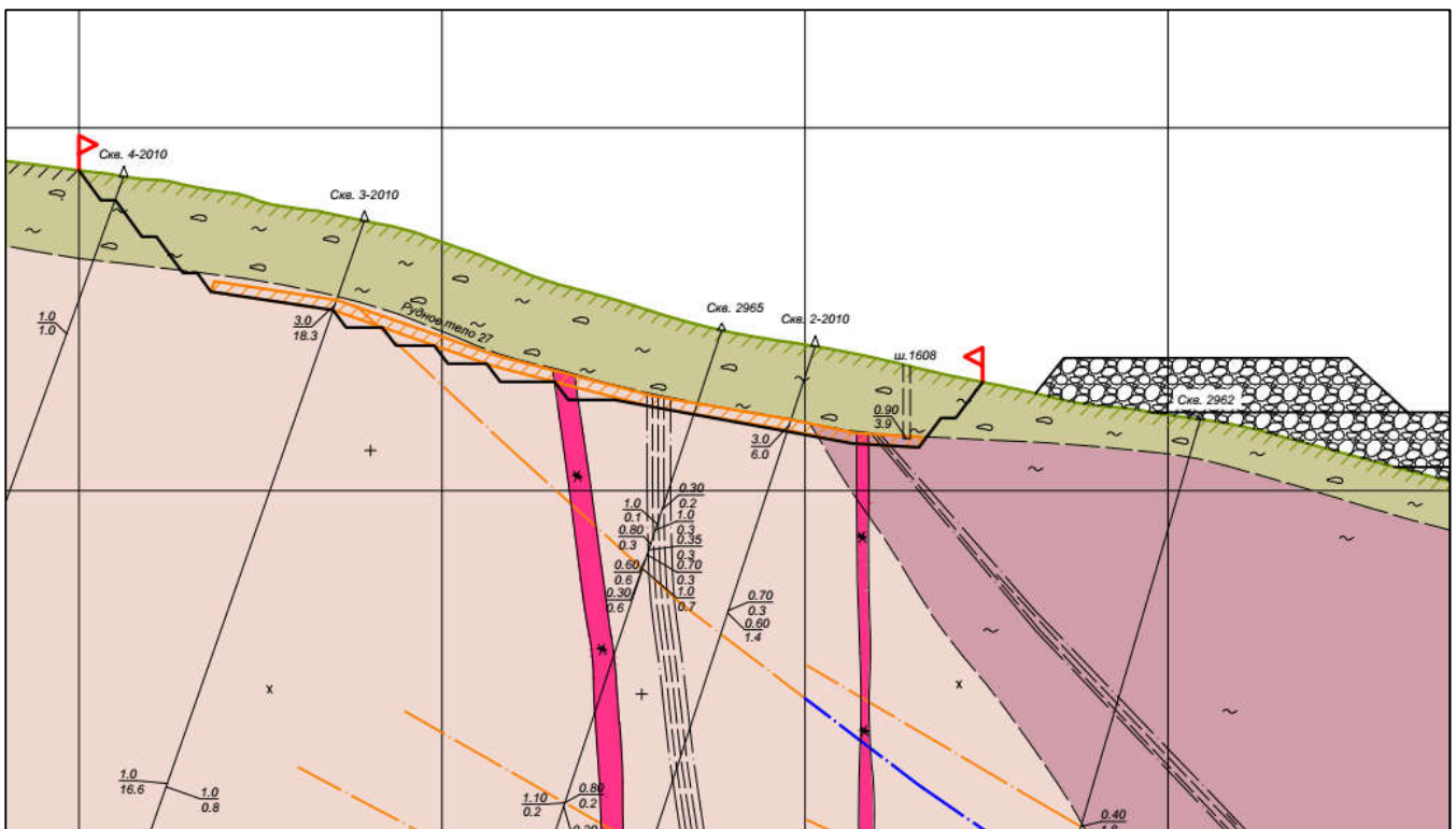
Рис. 2. Разрез рудного тела 27 и карьера для его отработки
